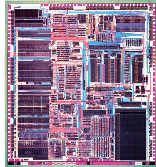
Intel Corporation, 1985. 229.000 transistores. Microprocesador (386™) [MoMA, Nueva York].
