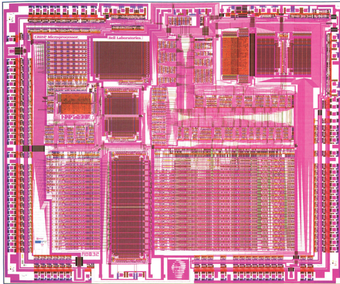
AT&T Bell Laboratories, 1986. 172.000 transistores. Microprocesador (CRISP).
