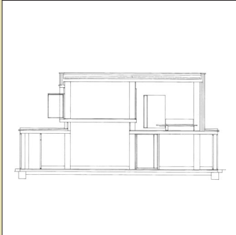
Centro Cultural en Canovelles. Barcelona, 1983-1986 Canovelles Cultural Centre. Barcelona, 1983-1986
